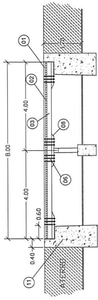
CORTE A-A LONGITUDINAL
