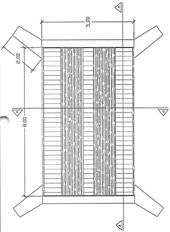
PLANTA - BAIXA
