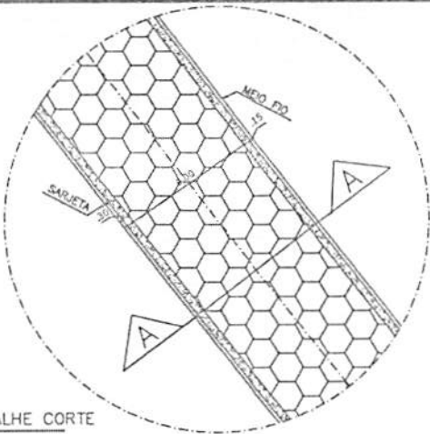
DETALHE 01 ESC: 1/75
