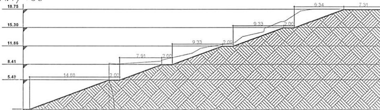
CORTE 02 ESCALA: 1/300
