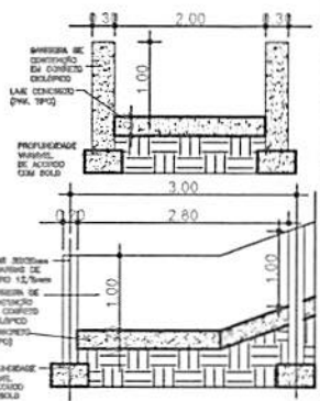
DETALHE 01 ESCALA: 1/50
