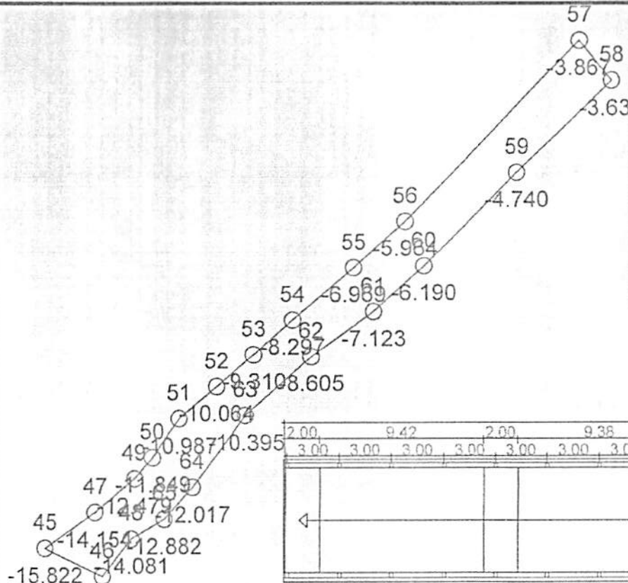
LOCAÇÃO 02 ESCALA: 1/150
