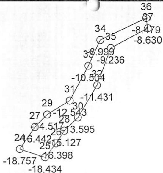
LOCAÇÃO 02 ESCALA: 1/150
