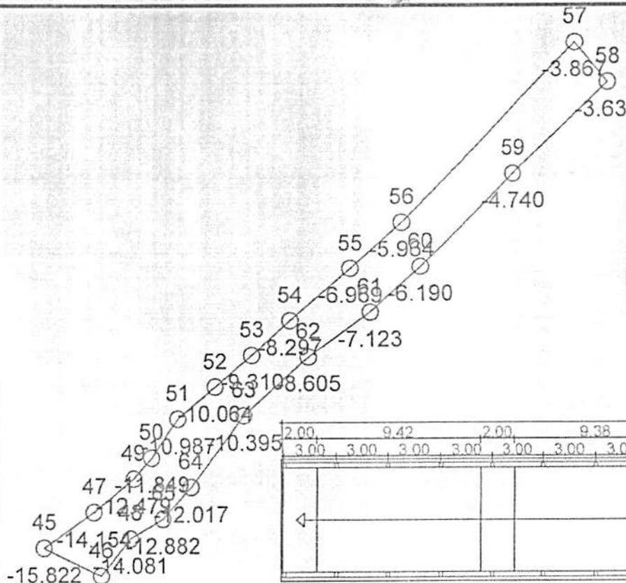
VISTA 02 ESCALA: 1/100
