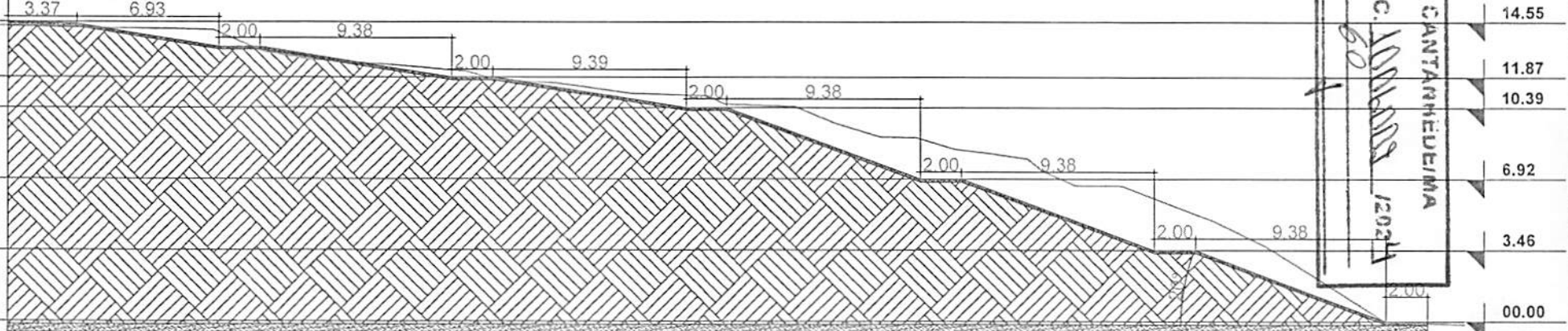
CORTE 01 ESCALA: 1/300
