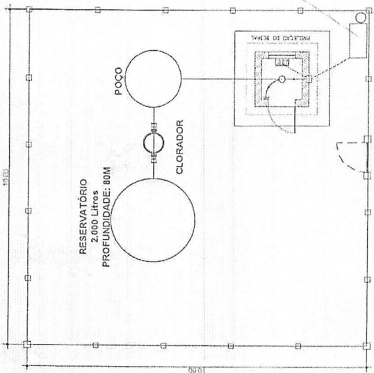
DET. POÇO Esc: 1/50
